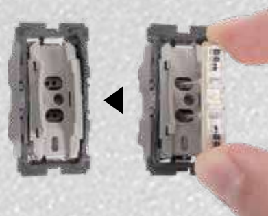
Illesse össze a két mechanizmust a kettős funkció létrehozásához. Illesze be a LED-et, ha szükséges (1)
