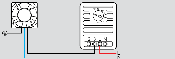
Ventilátor
