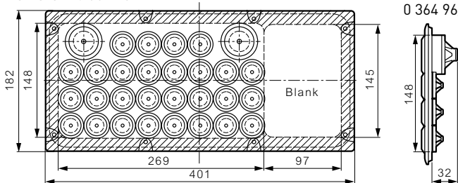
Kat. szám 0 364 96
