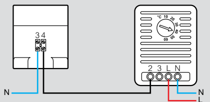
Ventilátor
