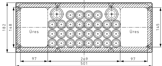
Kat. szám 0 364 97
