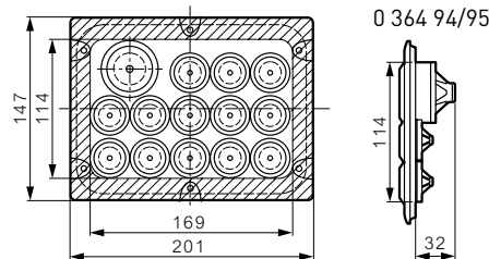
Kat. szám 0 364 94
