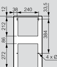
Kat. szám 0 353 47
