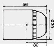
110KN E 27 Fassung, glatt mit Metallnippelgewinde M10 x 1 und Madenschraube
