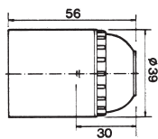
120 E 27 Schraubfassung mit Isogewinde M10 x 1 Verdrehungsschutz außen Bohrung für Madenschraube 2,5x10
