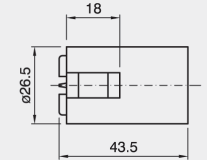
140 S E 14 Fassung, glatt mit Steckklemmen
