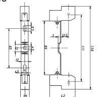
417/S 50 Halogenfassung R 7s (DRDG) für Halogen/LEDstäbe 117 mm mit Anschlussleitung 250 mm -Silikon ... T180° -Teflon ... T250°
