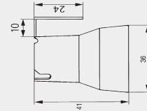
922 E 14 Porzellanfassung mit Innenbügel
