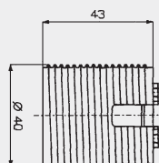
120 S E 27 Schraubmantelfassung mit Steckklemmen
