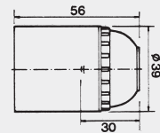
110MS E 27 Fassung, glatt mit Isogewinde M10 x 1 Verdrehungsschutz außen mit eingedrehter Madenschraube
