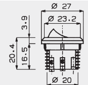
6273/6274 Wippschalter rund inkl. Klemmring 2 A / 250V
