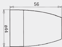
913 E 27 Porzellanfassung dreiteilig mit Metallplatte, Maden- schraube und Erde M10 x 1 M13 x 1 G3/8
