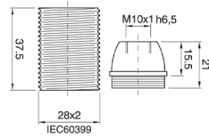
141 S E 14 Fassung Außengewinde kurz mit Steckklemmen
