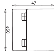
915 E 27 Porzellanfassung zweiteilig, Bodenbefestigung Lochabstand 35mm
