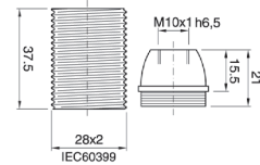
140 S E 14 Fassung, glatt mit Steckklemmen
