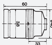
2000 N E 27 Zugschalterfassung glatt, Metall mit Erdungsklemme mit Metallnippelgewinde M10 x 1 und Madenschraube
