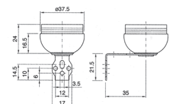
110B2A E 27 Fassung mit Außenbügel, glatt mit oder ohne Erdungsklemme Lochabstand 12 mm, Loch 3,2 mm
