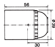
120MS E 27 Schraubfassung mit Isogewinde M10 x 1 Verdrehungsschutz außen mit eingedrehter Madenschraube
