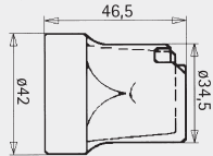
910 E 27 Porzellanfassung Bodenbefestigung 18 mm Loch-abstand
