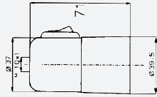
1100 Z E 27 Zugschalterfassung glatt, Thermoplast mit Metallnippelgewinde M10 x 1 und Madenschraube
