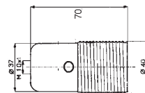
1200 Z E 27 Zugschalterfassung Außengewindemantel Thermoplast mit Metallnippelgewinde M10 x 1 und Madenschraube
