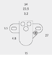
6237 Zug-Serienschalter 2 A/250 V AC
