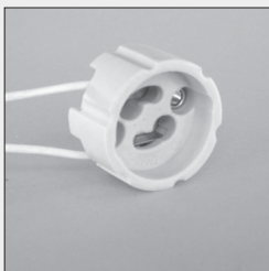
12600Z Hochvolt Halogenfassung GZ10 2A/250V, GU/GZ Anschlussleitung 250 mm
