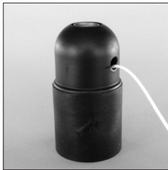
1100 Z E 27 Zugschalterfassung glatt, Thermoplast mit Metallnippelgewinde M10 x 1 und Madenschraube
