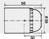
110KNL E 27 Fassung, glatt mit Metallnippelgewinde M10 x 1 und Madenschraube, Kappe mit seitlicher Kabeleinführung
