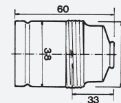
2002 N E 27 Zugschalterfassung Außengewindemantel, Metall mit Erdungsklemme und Metallnippelgewinde M10 x 1 und Madenschraube
