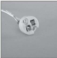
407 Niedervolt-Halogenfassung Universal G 4 - GX 5,3 - GY 6,35 - 15 ... Leitung Silikon 125 mm
