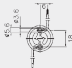
417/00 Halogenfassung R 7s mit Anschlussleitung 250 mm -Silikon ... T180° -Teflon ... T250°
