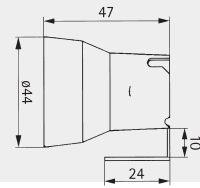
915 E 27 Porzellanfassung zweiteilig, Bodenbefestigung Lochabstand 35mm
