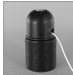
1200 Z E 27 Zugschalterfassung Außengewindemantel Thermoplast mit Metallnippelgewinde M10 x 1 und Madenschraube
