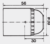
110 E 27 Fassung, glatt mit Isogewinde M10 x 1 Verdrehungsschutz außen Bohrung für Madenschchraube 2,5x10
