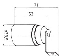
5010 BI ... mit Innenbügel 5010 BA ... mit Außenbügel E 27 Fassung, glatter Mantel Lochabstand 12mm; Loch 3,2mm
