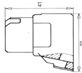
920 E 14 Porzellanfassung mit Befestigungskragen
