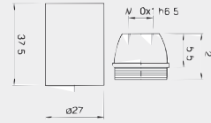
150KMS E 14 Schraubfassung mit Isogewinde M10 x 1 Verdrehungsschutz außen mit eingedrehter Madenschraube
