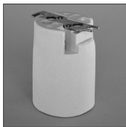
940 E 40 Porzellanfassung Bodenbefestigung Lochabstand 55 mm
