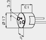
407 Niedervolt-Halogenfassung Universal G 4 - GX 5,3 - GY 6,35 - 15 ... Leitung Silikon 125 mm
