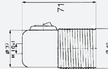
1200 D E 27 Druckschalterfassung Außengewindemantel Thermoplast mit Metallnippelgewinde M10 x 1 und Madenschraube
