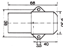
2414 D E 14 Winkelfassung mit Druckschalter (unmontiert)
