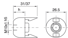
150 S E 14 Schraubfassung mit Steckklemmen
