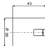
115 N E 27 Rastkappe mit Metallnippel M10 x 1 und Madenschraube
