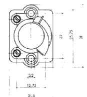
6237 Zug-Serienschalter 2 A/250 V AC
