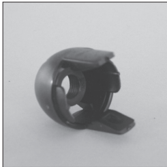
190 E 14 Rastkappe mit Isogewinde M10 x 1
