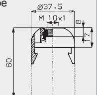
115 E 27 Rastkappe mit Isogewinde M10 x 1
