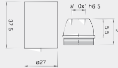
150K E 14 Schraubfassung mit Isogewinde M10 x 1 Verdrehungsschutz außen Bohrung für Madenschraube 2,5x10
