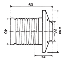
2260M E 27 Pendelfassung Metall mit Nippel M10 x 1 und Madenschraube
