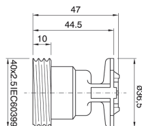
111 S E 27 Fassung naturfarben Außengewinde kurz, mit Steckklemmen
